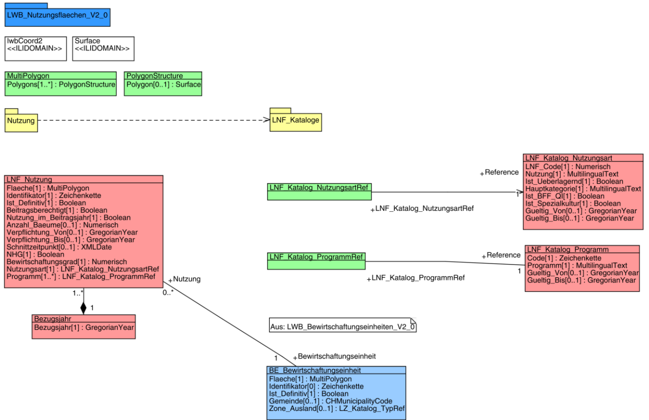
Abbildung 10: UML Diagramm Nutzungsflächen (inkl. BFF QI)
