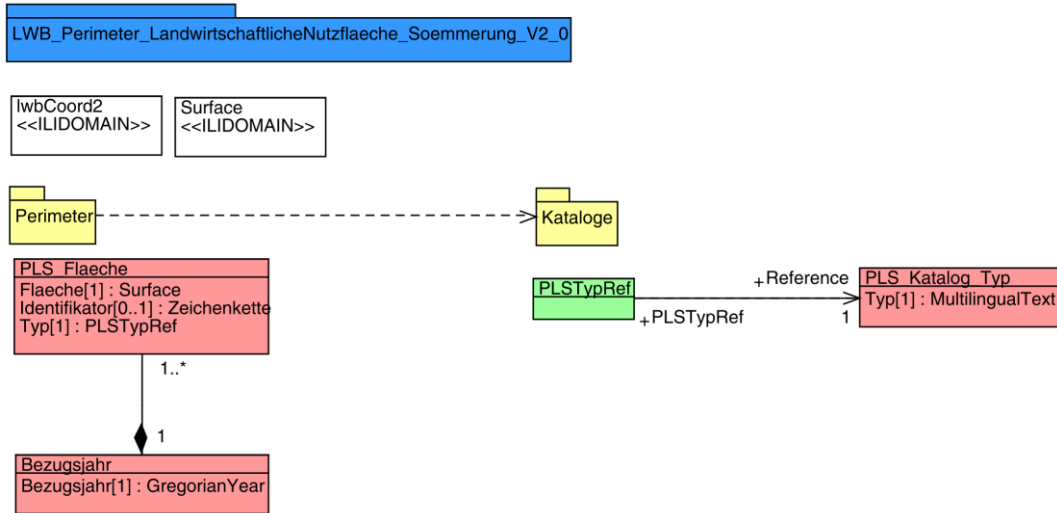
Abbildung 8: UML Diagramm Perimeter Landwirtschaftliche Nutzfläche und Sömmerungsflächen
